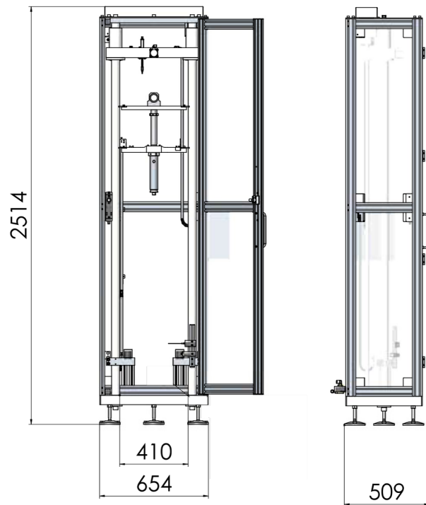
DW750 - Dimensions
